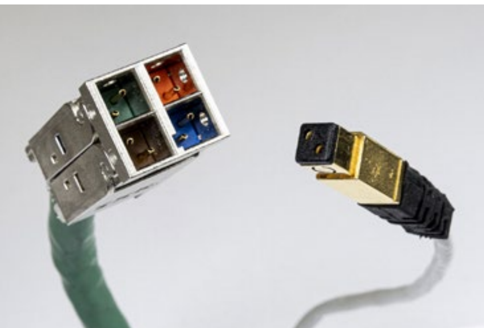
Avec MMCpro, vous êtes prêts pour le Single Pair Ethernet (SPE).
