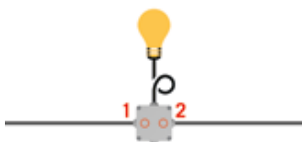
Installation électrique classique: au moins 2 points de contact avec pertes de résistance sur la ligne d'alimentation par dérivation.
